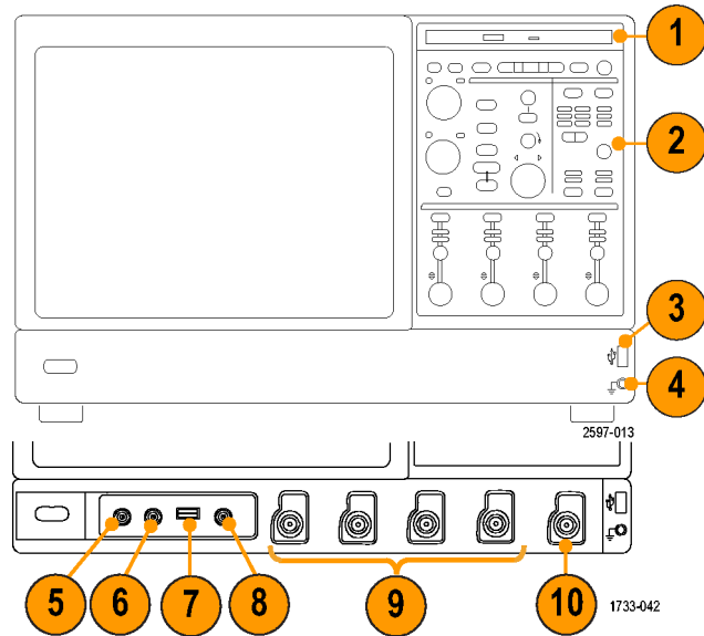
DPO7000C 系列
